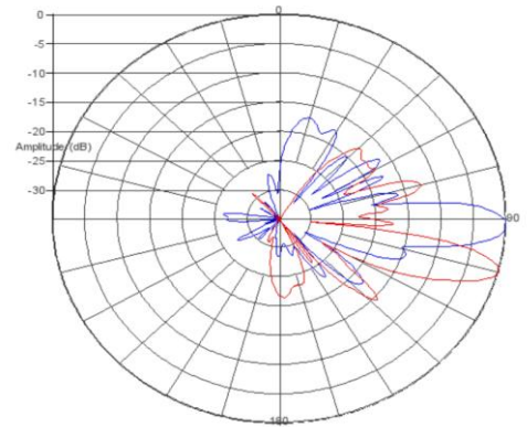
Vertical Patterns (2°, 15°)
