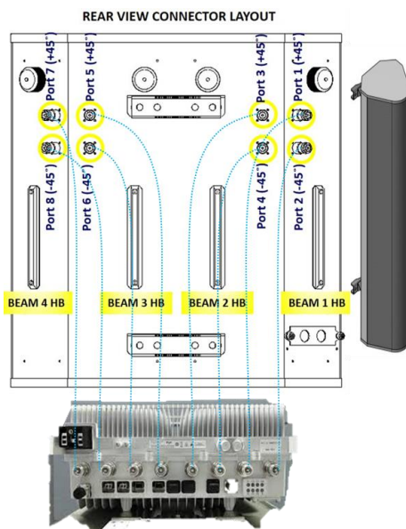
8T8R-RRH-2
