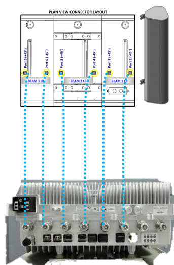
8T8R-RRH-2
