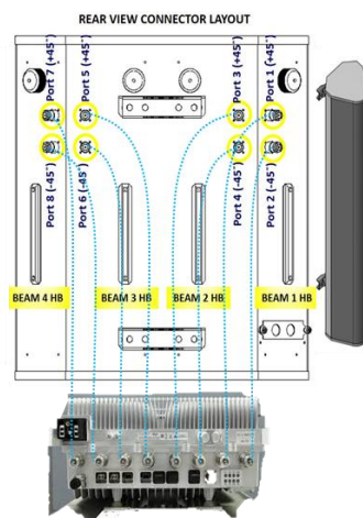
8T8R-RRH-2
